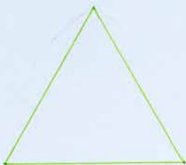
triunghi echilateral
