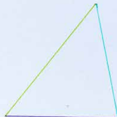
triunghi oarecare
