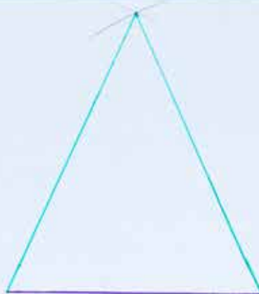
triunghi isoscel
